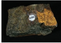
Volcanic breccia
