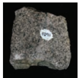
Granodiorite
